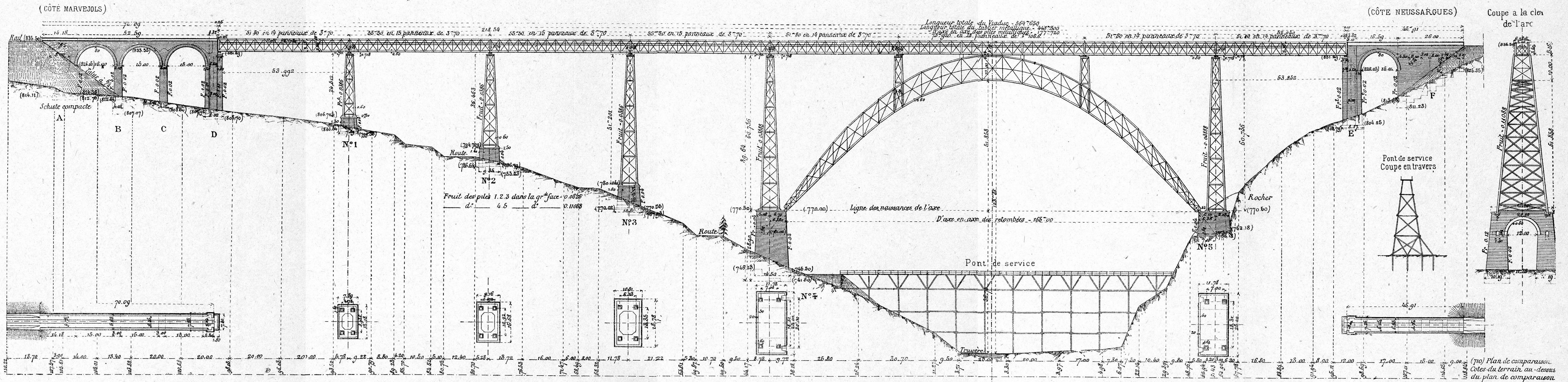
FIG. 374. — Viaduc de Garabit achevé. Vue du pont de service.
