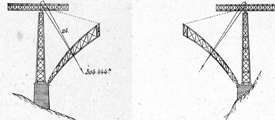
FIG. 373. — Viaduc de Garabit. Montage (4° phase).
