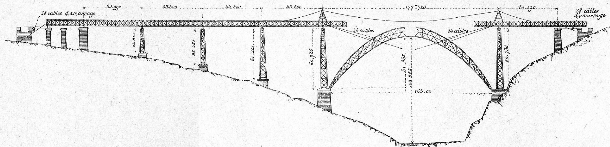
FIG. 372. — Viaduc de Garabit. Ensemble de la disposition des amarrages pendant le montage.
